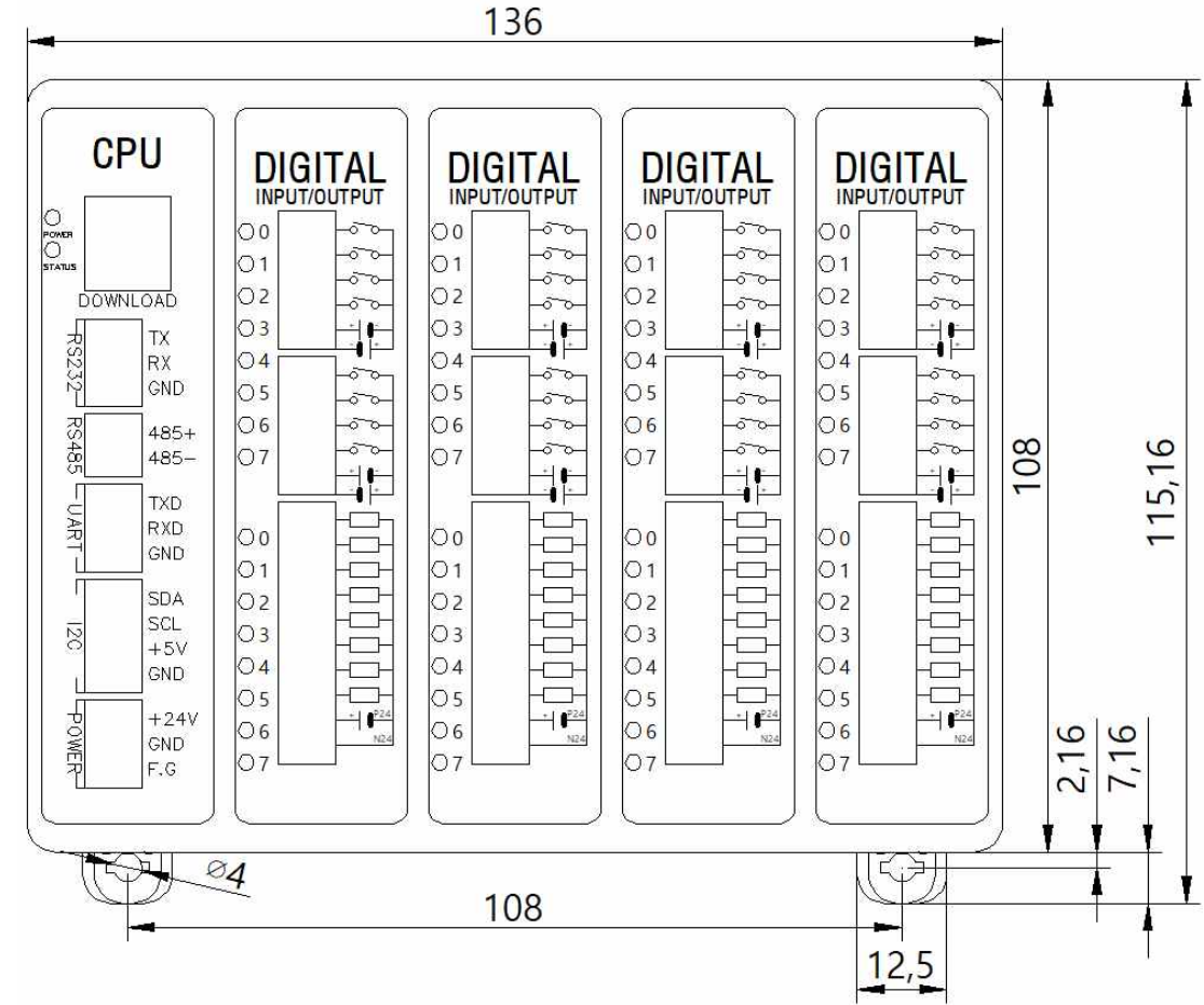
□ DIMENSION ( 딘 레일 : 35mm )
