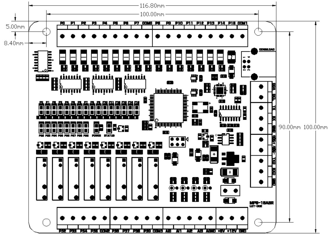
□ DIMENSION ( PCB / 단레일 사용하지 않을 경우 )
