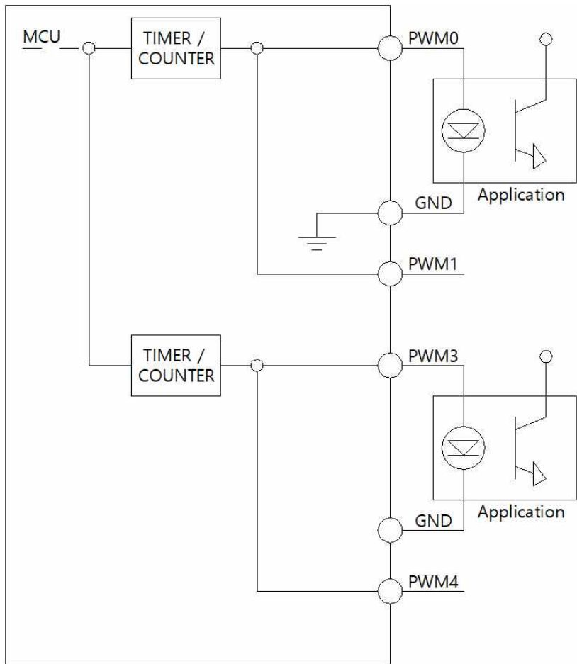
PWM(Pulse Width Modulator) 펄스의 DUTY와 WIDTH 관계
