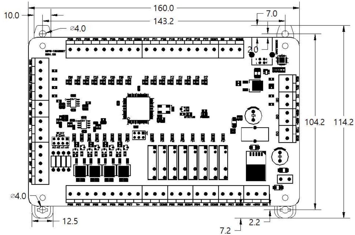
□ DIMENSION ( 클립 열었을 때 / 단 레일 체결 후 )
