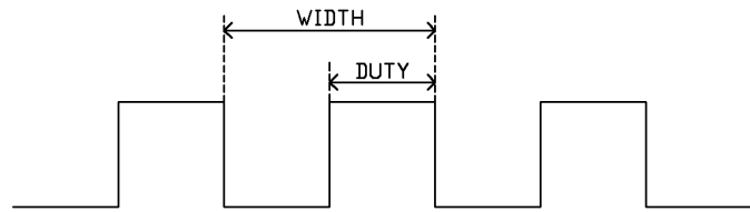
[ PWM 펄스의 DUTY와 WIDTH의 관계 ]
